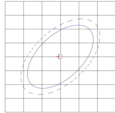
CIE1931色品图
